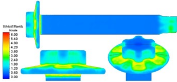
Şekil. 5. Marka zımbasının revize edilmesi sonucu simülasyondan alınan yarı mamul ürün formu.
