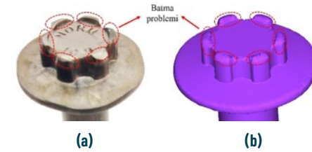
Şekil 2. Kafa formunda meydana gelen batma; (a) üretim, (b) simülasyon.
