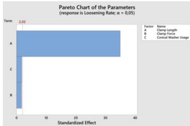
Fig. 6. Pareto chart of parameter effects.
