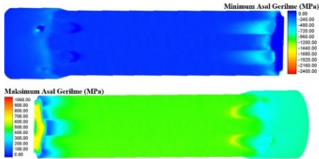
Şekil. 6. Dövme sonunda zımba formunda oluşan minimum asal gerilme değerleri.
