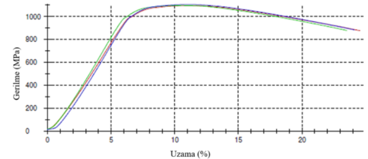
Şekil 6. Çekme testinde gerilme-uzama ilişkisi.
