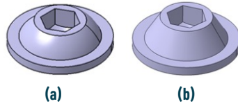
Şekil 3. Bağlantı elemanı kafa formu; (a) DIN EN ISO 7380-2 (b) revize tasarım.
