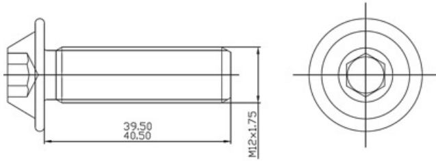
Şekil 1. M12x1,75x40 (DIN ISO EN 7380-2).
