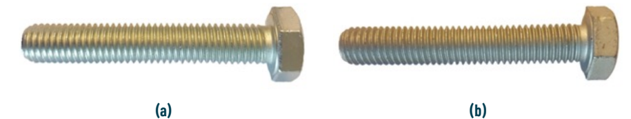
Fig. 1. Specimens; a) Zn-Cr 3 b) Zinc flake.
