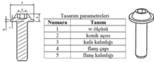
Şekil 2. Ürün tasarımında incelenen tasarım parametreleri.
